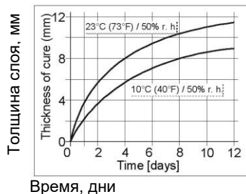
Диаграмма 1: скорость отверждения SikaTack® Go!.
